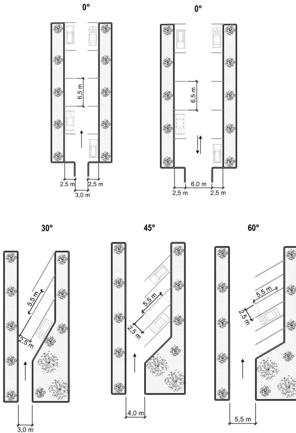
Figure 7-8 - Dimensions relatives aux cases de stationnement, aux allées d'accès et aux allées de circulation
