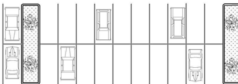
Figure 7-7 - Aménagement des îlots de verdure PROPOSITION "D"
