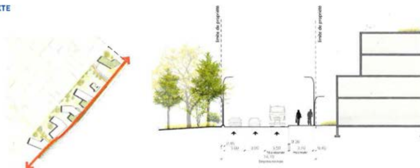
Fig. 132. Coupe, Rue collectrice mixte
