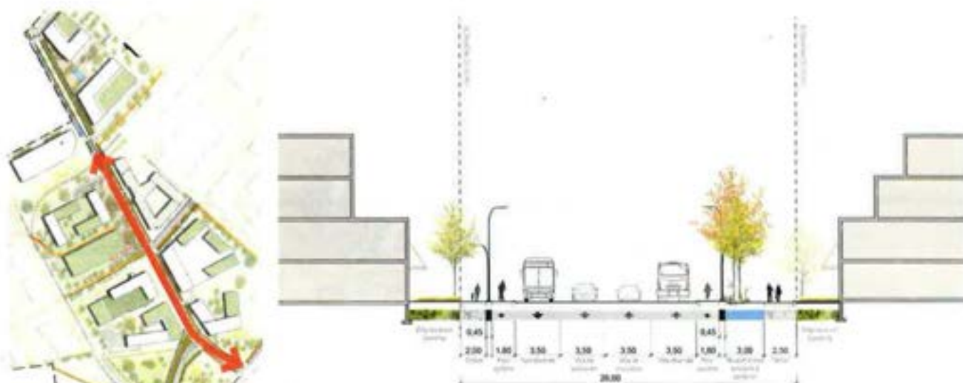
Fig. 167. Coupe, Boulevard Montcalm entre le boulevard de l'Industrie et la rue partagée
