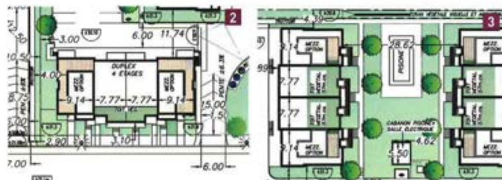
Fig. 232. [2] et [3] Extraits du plan d'implantation des Duplex et Triplex du Square Candiac.
