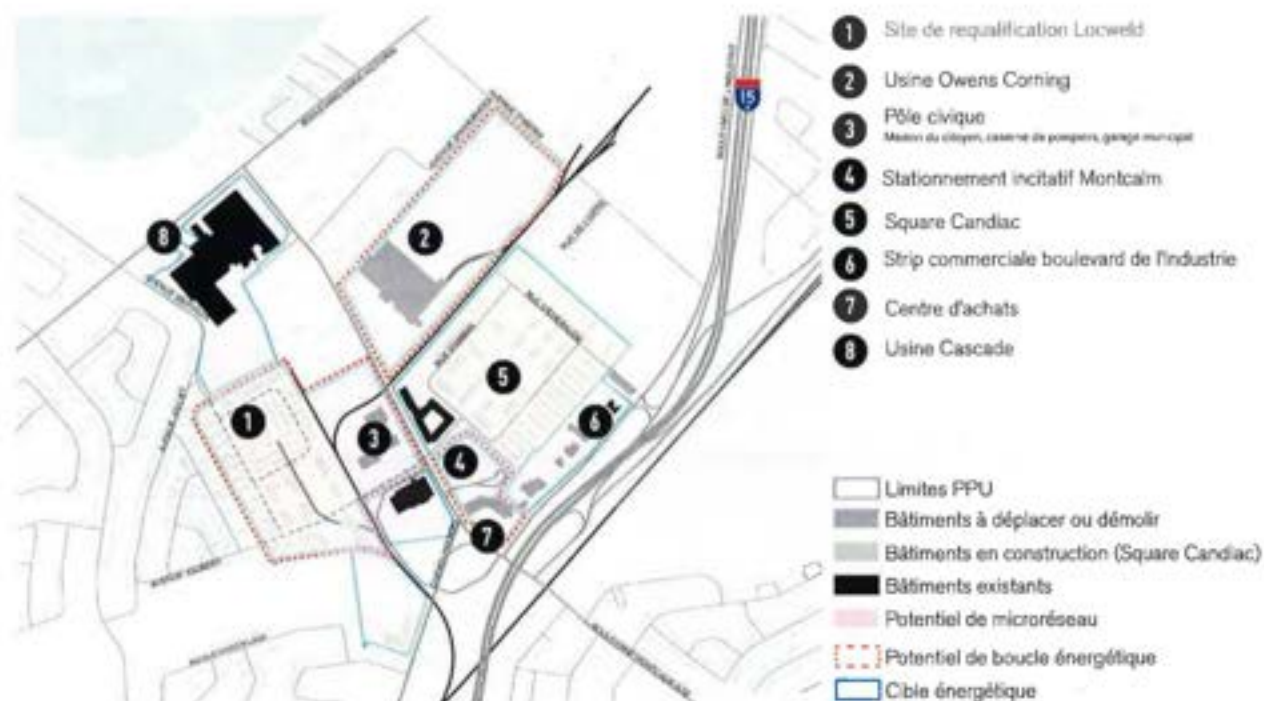
Fig. 146. Implantation des stratégies énergétiques (Source: Ville de Candiac)
