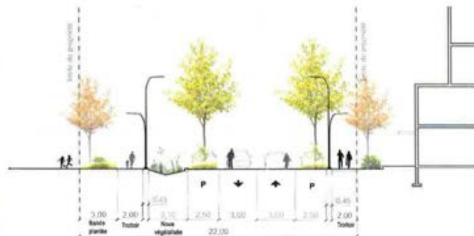
Fig. 171. Coupe, Rue partagée
