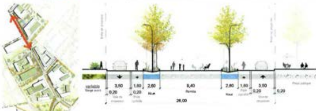
Fig. 115. Coupe, Boulevard Montcalm la voie de chemin de fer et la rambla
